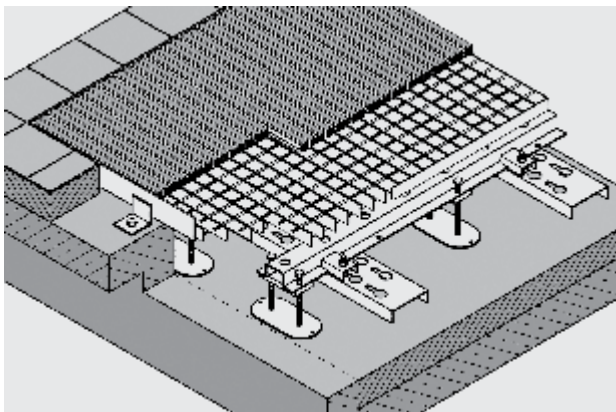
Unterkonstruktion
