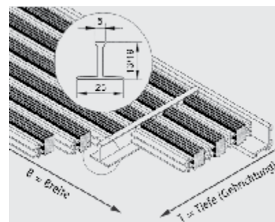
Mattentrennprofil
