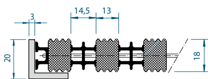
Plaingard G
