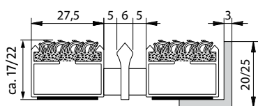
Portagard IK
