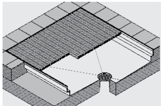
Schmutzfangwanne PortaDrain
