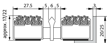
Portagard IK
